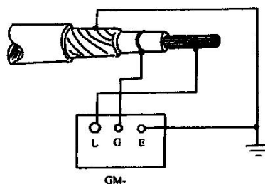
屏蔽电缆绝缘测试接线图
